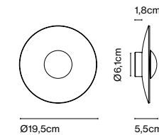
Ginger 20 C IP65*
